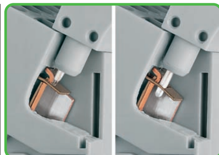
A = Подпружиненный контакт центрального модуля B = Оконечный модуль с жестким контактом
